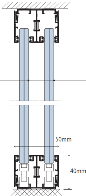
DOPPIO-VETRO DOUBLE-GLAZING DOUBLE-VITRAGE
