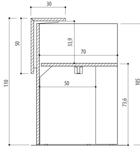
SEZIONE VERTICALE MODULI RECEPTION vertical section of reception modules
