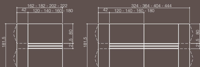
Scrivanie con cassettiere complanari Desks with desk-height pedestals
