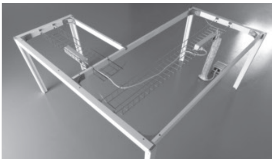
Horizontal wiring grids Griglie per cablaggio orizzontale _ Grille pour le câblage horizontal _ Gitterkorb zur Aufnahme von Kabeln Rejillas para electrificación horizontal
